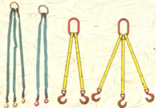
Multileg Slings
